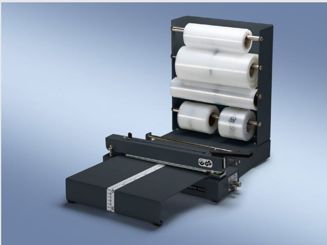
243 M AVEC TABLE À ENFICHER ET MAGASIN À BOBINES
